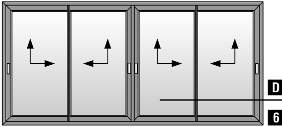
Τετράφυλλο επάλληλο ανασυρόμενο παράθυρο (κοπή 90°) Four sash parallel lift & slide window (90° cutting)
