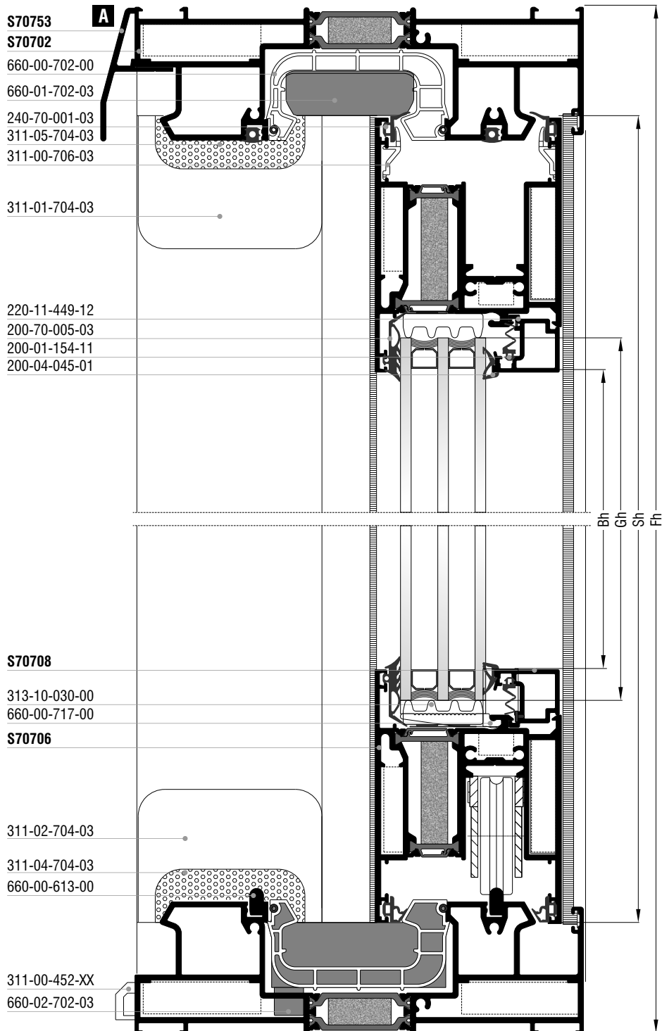
Τετράφυλλο επάλληλο ανασυρόμενο παράθυρο Four sash parallel lift & slide window
