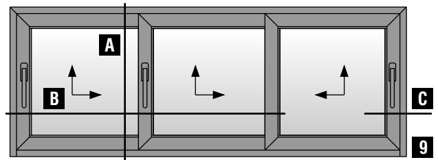
Τρίφυλλο επάλληλο ανασυρόμενο παράθυρο με χρήση τριπλού οδηγού & χαμηλού οδηγού S70762 Three sash parallel lift & slide window with triple frame guide & S70762 short frame guide use
