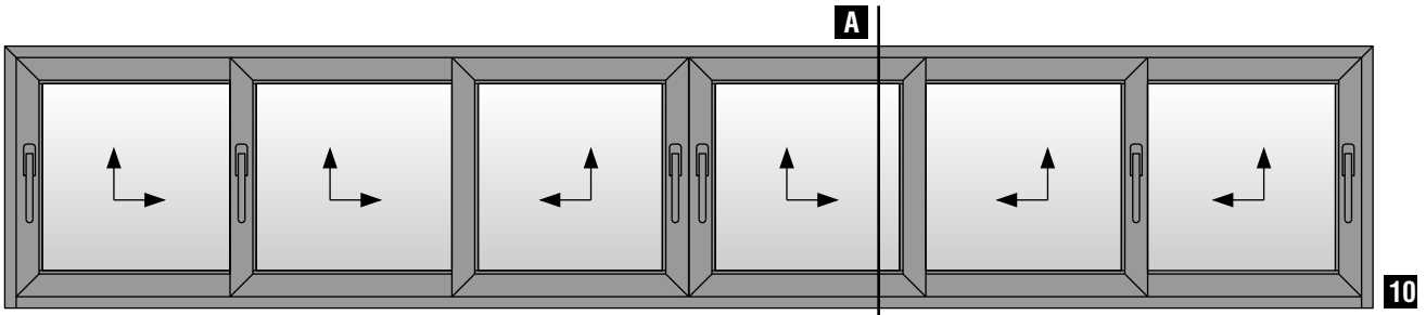
Εξάφυλλο επάλληλο φιλητό ανασυρόμενο παράθυρο με χρήση τριπλού οδηγού & χαμηλού οδηγού S70762 Six sash parallel meeting stile lift & slide window with triple frame guide & S70762 short frame guide use
