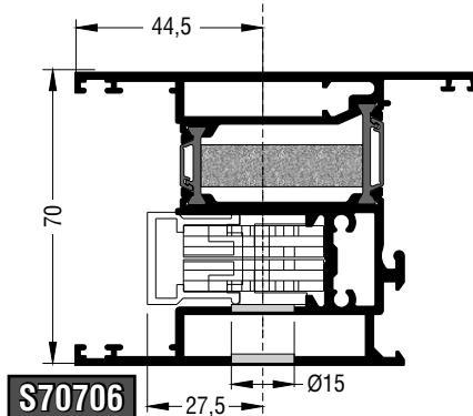
Κατεργασία καρέ | Square machining
