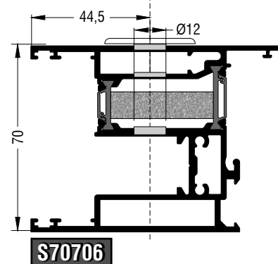
Κατεργασία ροζέτας | Rosette machining
