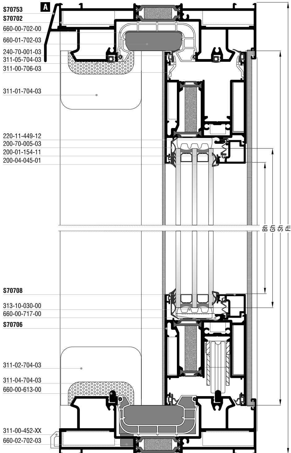
Τετράφυλλο επάλληλο ανασυρόμενο παράθυρο (κοπή 90°) Four sash parallel lif & slide window (90° cutting)
