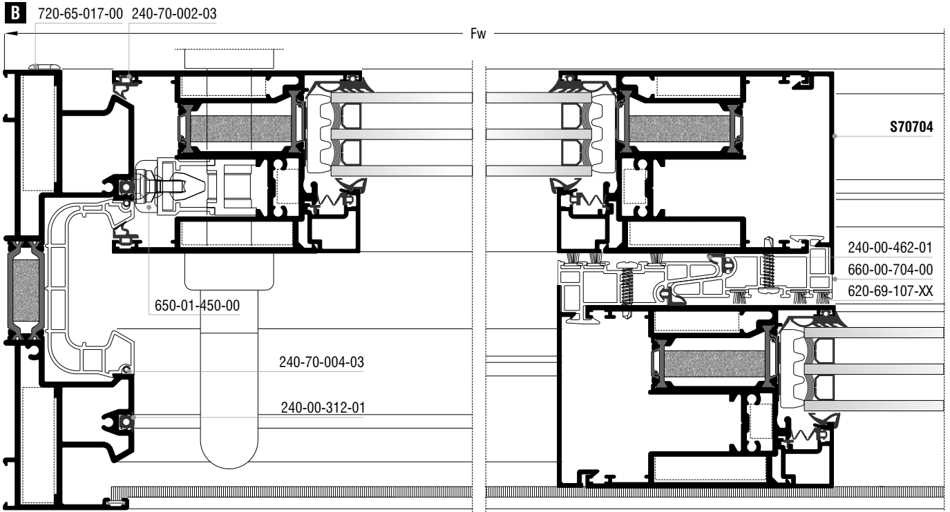
Τετράφυλλο επάλληλο ανασυρόμενο παράθυρο Four sash parallel lift & slide window
