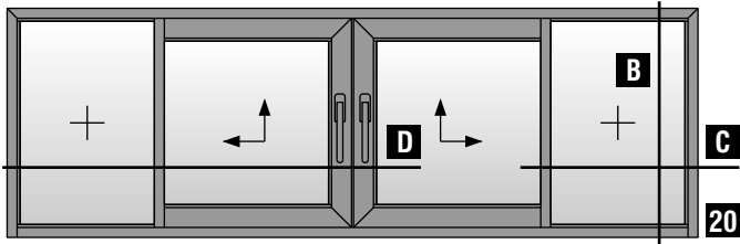
Δίφυλλο φιλητό ανασυρόμενο με σταθερά Two sash meeting stile lift & slide with fixed
