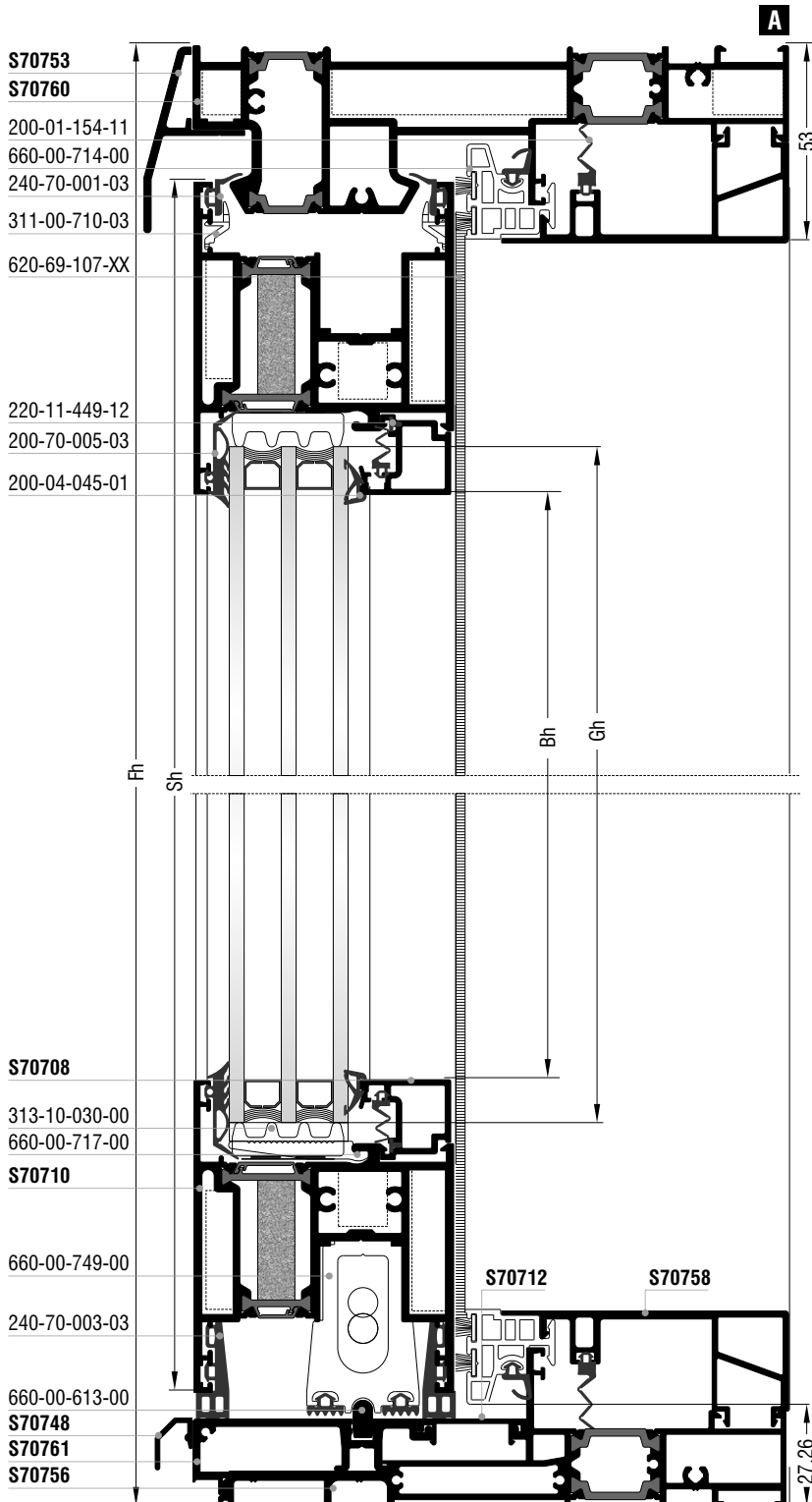
Δίφυλλο φιλητό ανασυρόμενο με σταθερά Two sash meeting stile lift & slide with fixed
