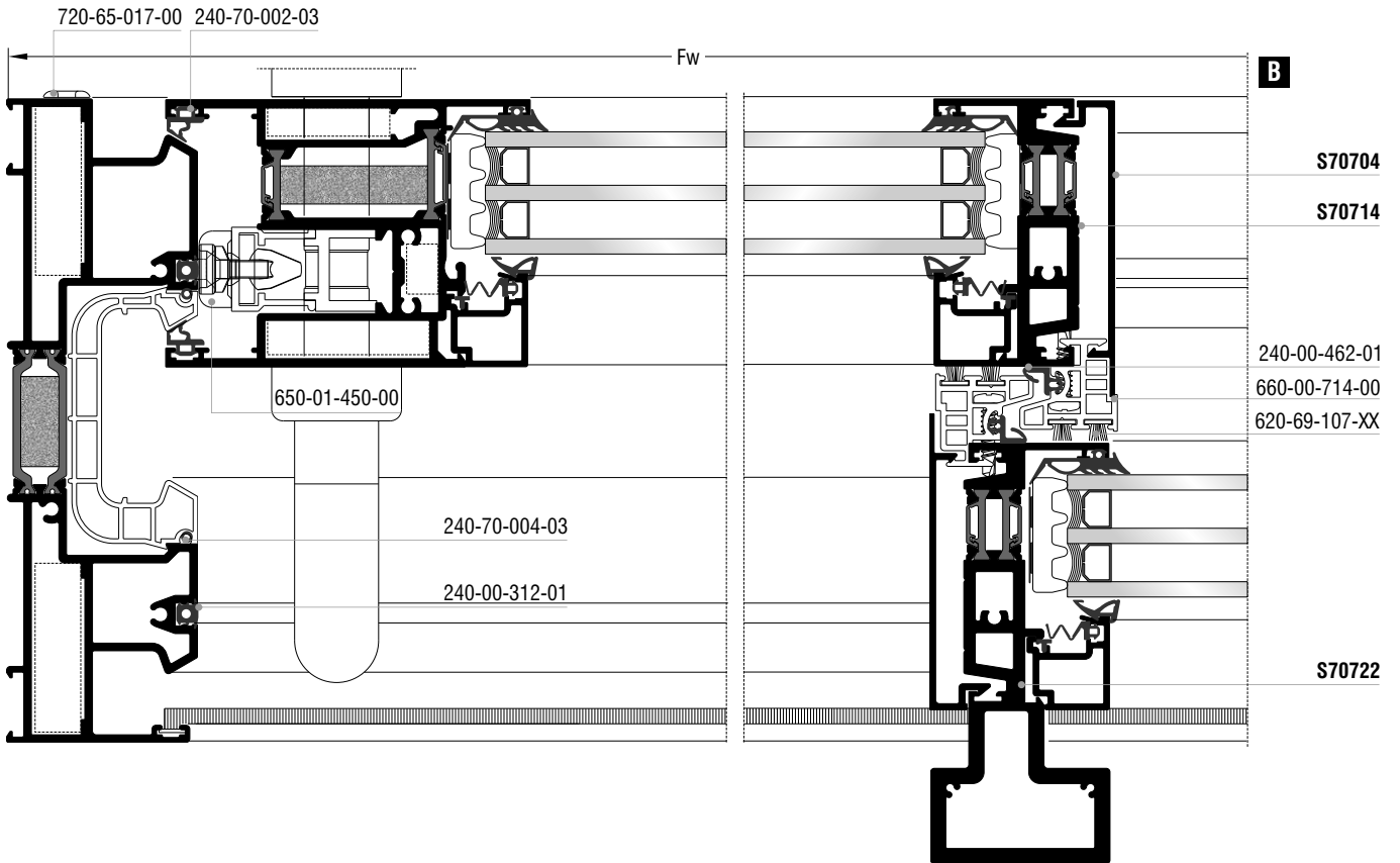
Τετράφυλλο επάλληλο ανασυρόμενο παράθυρο (κοπή 90°) Four sash parallel lif & slide window (90° cutting)
