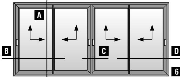
Τετράφυλλο επάλληλο ανασυρόμενο παράθυρο (κοπή 90°) Four sash parallel lift & slide window (90° cutting)
