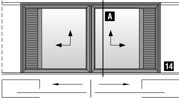
Δίφυλλο φιλητό χωνευτό ανασυρόμενο παράθυρο με παντζούρι Two sash meeting stile pocket lift & slide window with shutter
