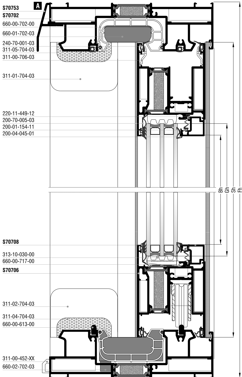
Δίφυλλο επάλληλο ανασυρόμενο παράθυρο Two sash parallel lift & slide window
