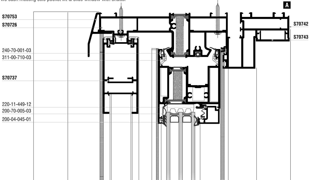
Δίφυλλο φιλητό χωνευτό ανασυρόμενο παράθυρο με παντζούρι Two sash meeting stile pocket lift & slide window with shutter
