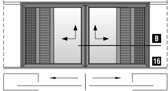
Δίφυλλο φιλητό χωνευτό ανασυρόμενο παράθυρο με σήτα και παντζούρι Two sash meeting stile pocket & slide window with fly-screen and shutter
