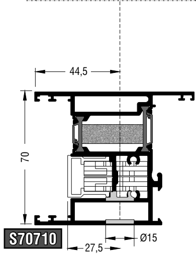
Κατεργασία καρέ | Square machining
