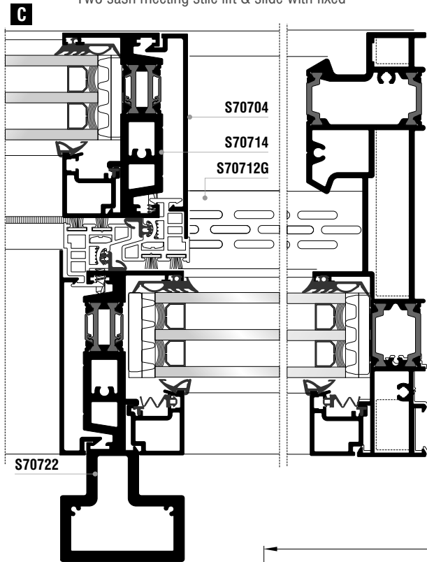
Δίφυλλο φιλητό ανασυρόμενο με σταθερά Two sash meeting stile lift & slide with fixed
