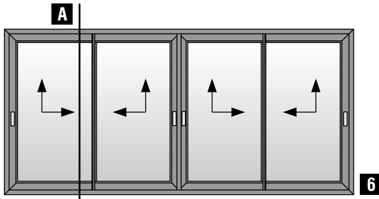
Τετράφυλλο επάλληλο ανασυρόμενο παράθυρο (κοπή 90°) Four sash parallel lif & slide window (90° cutting)
