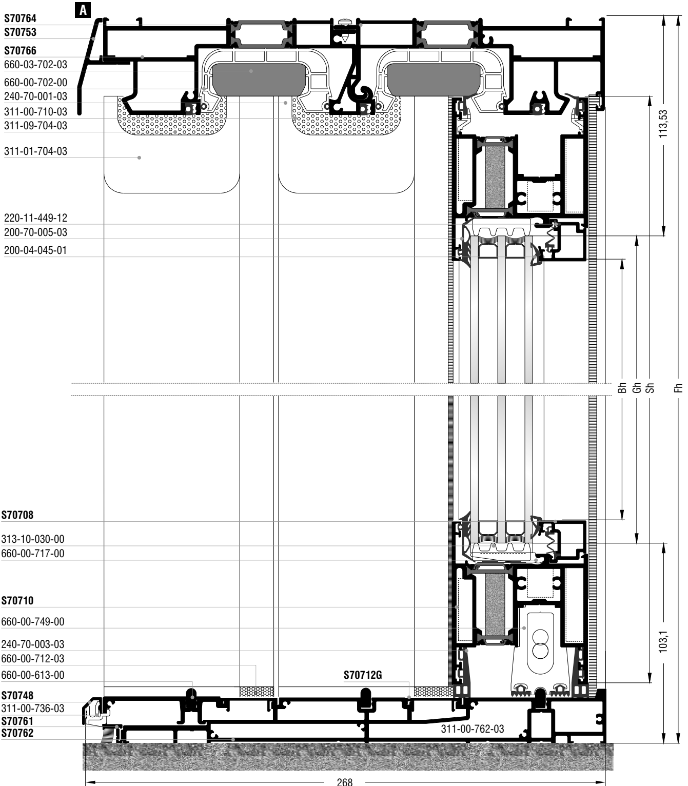
Εξάφυλλο επάλληλο φιλητό ανασυρόμενο παράθυρο με χρήση τριπλού οδηγού & χαμηλού οδηγού S70762 Six sash parallel meeting stile lift & slide window with triple frame guide & S70762 short frame guide use
