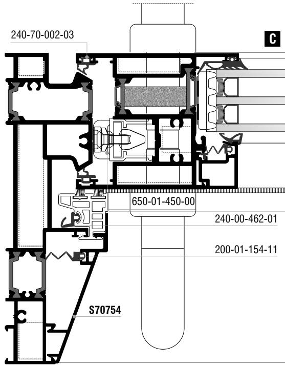
Δίφυλλο ανασυρόμενο με σταθερό | Two sash lift & slide with fixed
