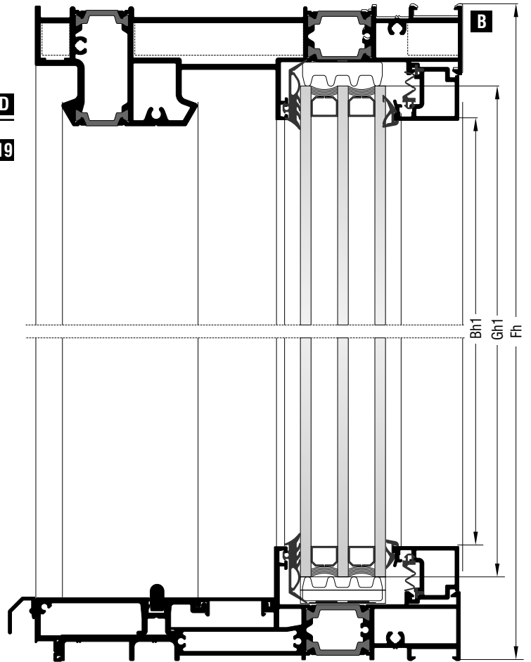
Δίφυλλο ανασυρόμενο με σταθερό | Two sash lift & slide with fixed
