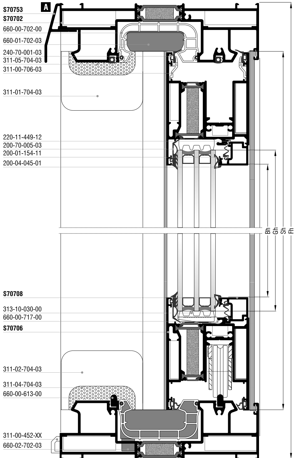
Δίφυλλο επάλληλο ανασυρόμενο παράθυρο (κοπή 90°) Two sash parallel lif & slide window (90° cutting)
