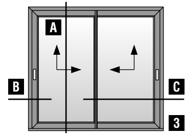
Δίφυλλο επάλληλο ανασυρόμενο παράθυρο με χρήση χαμηλού οδηγού S70720 (κοπή 90°) Two sash parallel lift & slide window with S70720 short frame guide use (90° cutting)
