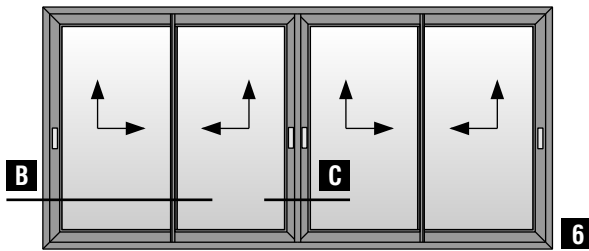
Τετράφυλλο επάλληλο ανασυρόμενο παράθυρο (κοπή 90°) Four sash parallel lif & slide window (90° cutting)
