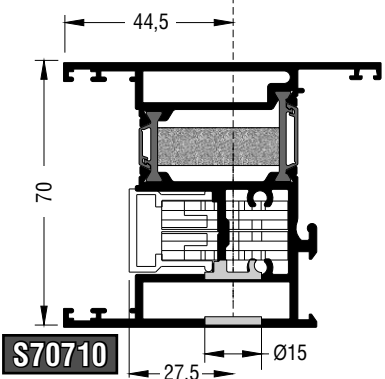
Κατεργασία καρτέ | Square machining
