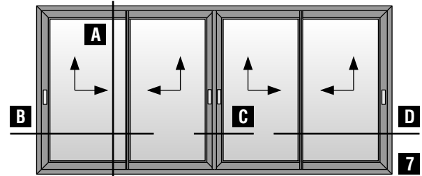
Τετράφυλλο επάλληλο ανασυρόμενο παράθυρο με χρήση χαμηλού οδηγού S70720 (κοπή 90°) Four sash parallel lift & slide window with S70720 short frame guide use (90° cutting)
