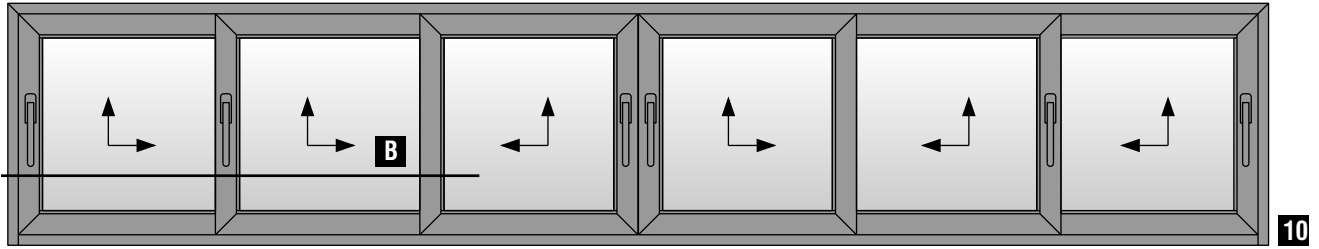
Εξάφυλλο επάλληλο φιλητό ανασυρόμενο παράθυρο με χρήση τριπλού οδηγού & χαμηλού οδηγού S70762 Six sash parallel meeting stile lift & slide window with triple frame guide & S70762 short frame guide use
